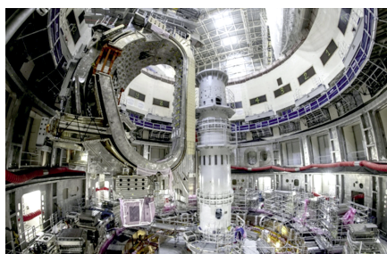
Figure 2 : Le 11 mai 2022, levée et installation du premier module de la chambre à vide (1.380 tonnes, l'équivalent de quatre Boeing 747 à pleine charge) dans la fosse du réacteur
