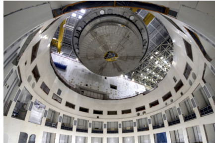
Figure 1 : Le 26 mai 2020, la base du cryostat, fabriquée en Inde, est descendue dans la fosse du tokamak
